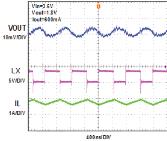
PWM MODE
