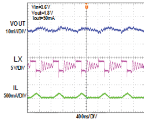
PFM MODE
