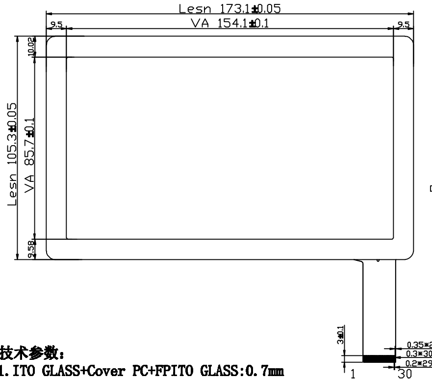
正视图
