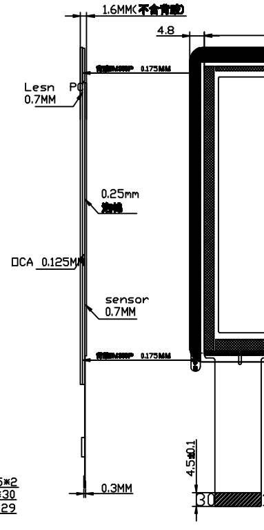
侧视图
