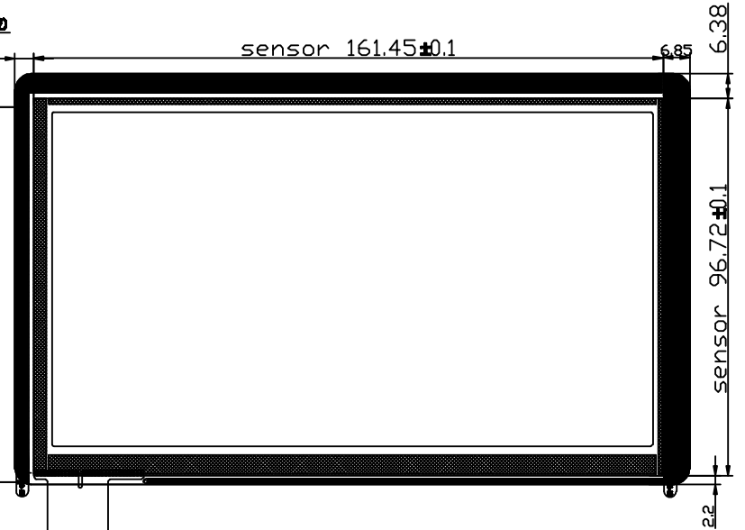
反视图
